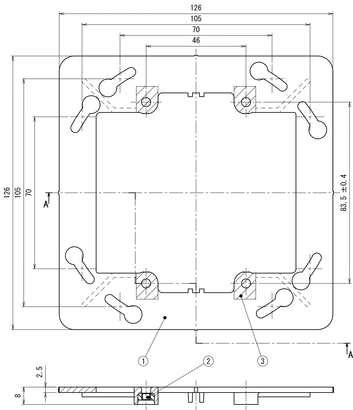
A-A断面図
